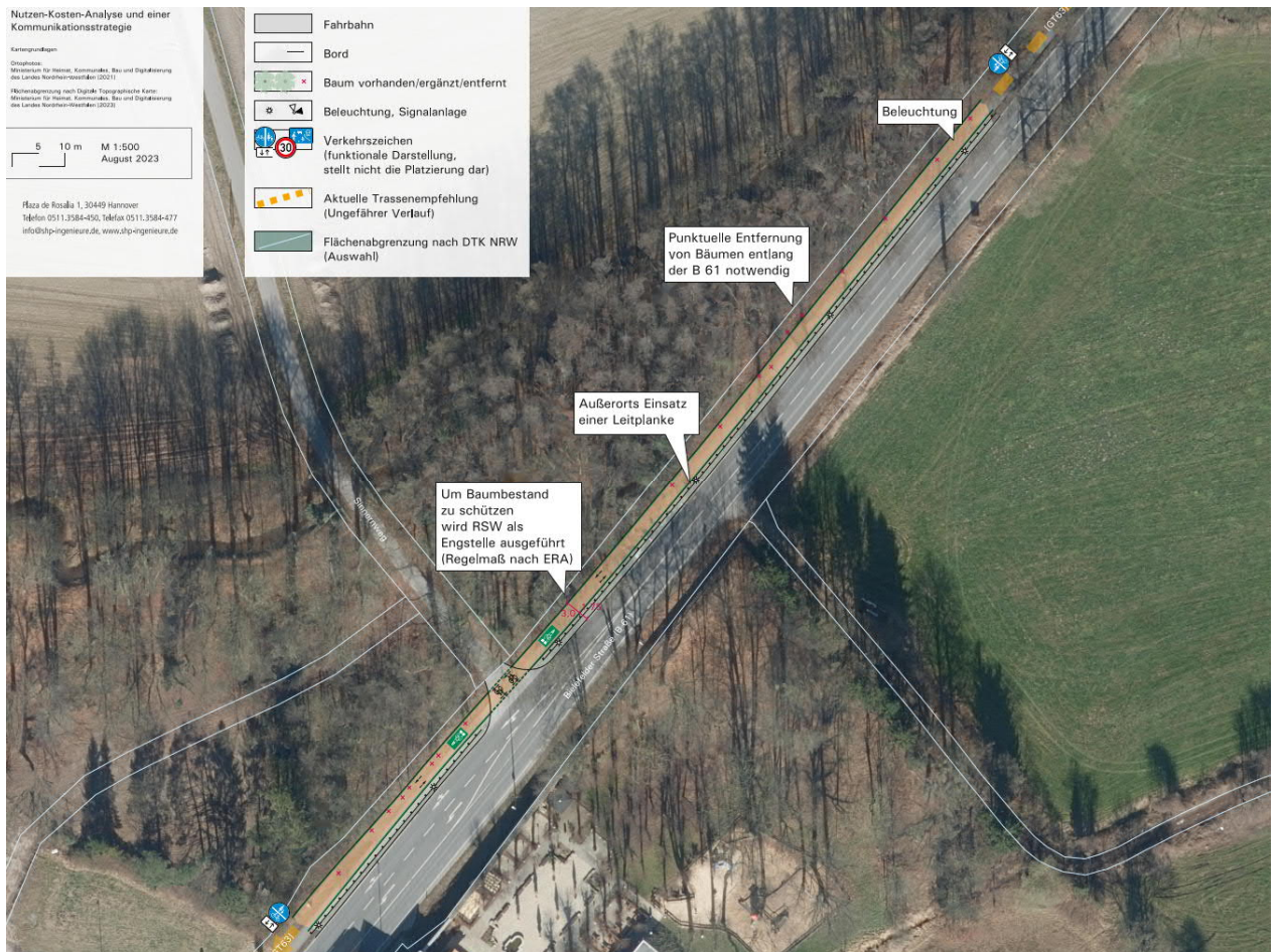
Abb. 38 Ausschnitt Planerische Lösung für einen Abschnitt an der B 61 zwischen Isselhorster Straße und Reiherbach/Stadtgrenze Gütersloh-Bielefeld, GT63 (nicht maßstäblich, Lageplan maßstabsgetreu und mit weiterführenden Informationen im Anhang)
