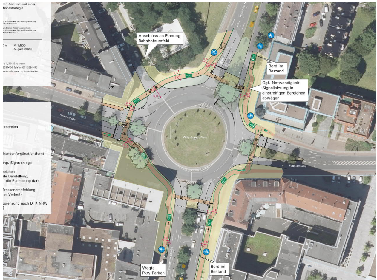
Abb. 45 Ausschnitt Planerische Lösung für den Willy-Brandt-Platz, BI111/BI56 (nicht maßstäblich, Lageplan maßstabsgetreu und mit weiterführenden Informationen im Anhang)
