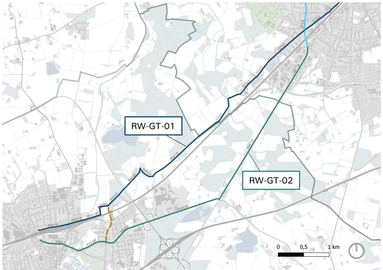
Abb. 19 Übersicht Trassenvarianten: Rheda-Wiedenbrück – Gütersloh (RW-GT)
