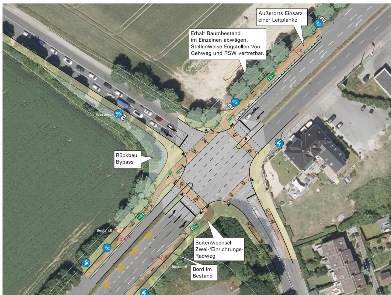
Abb. 47 Ausschnitt Planerische Lösung für den KP Herforder Straße/Talbrückenstraße, BI59/BI61 (nicht maßstäblich, Lageplan maßstabsgetreu und mit weiterführenden Informationen im Anhang)
