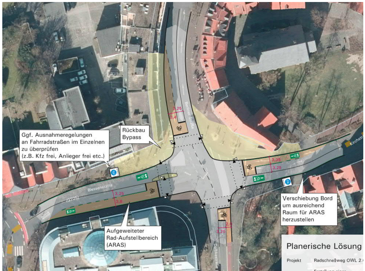
Abb. 32 Ausschnitt Planerische Lösung für den KP Blessenstätte/Kirchstraße/Berliner Straße, GT05 (nicht maßstäblich, Lageplan maßstabsgetreu und mit weiterführenden Informationen im Anhang)
