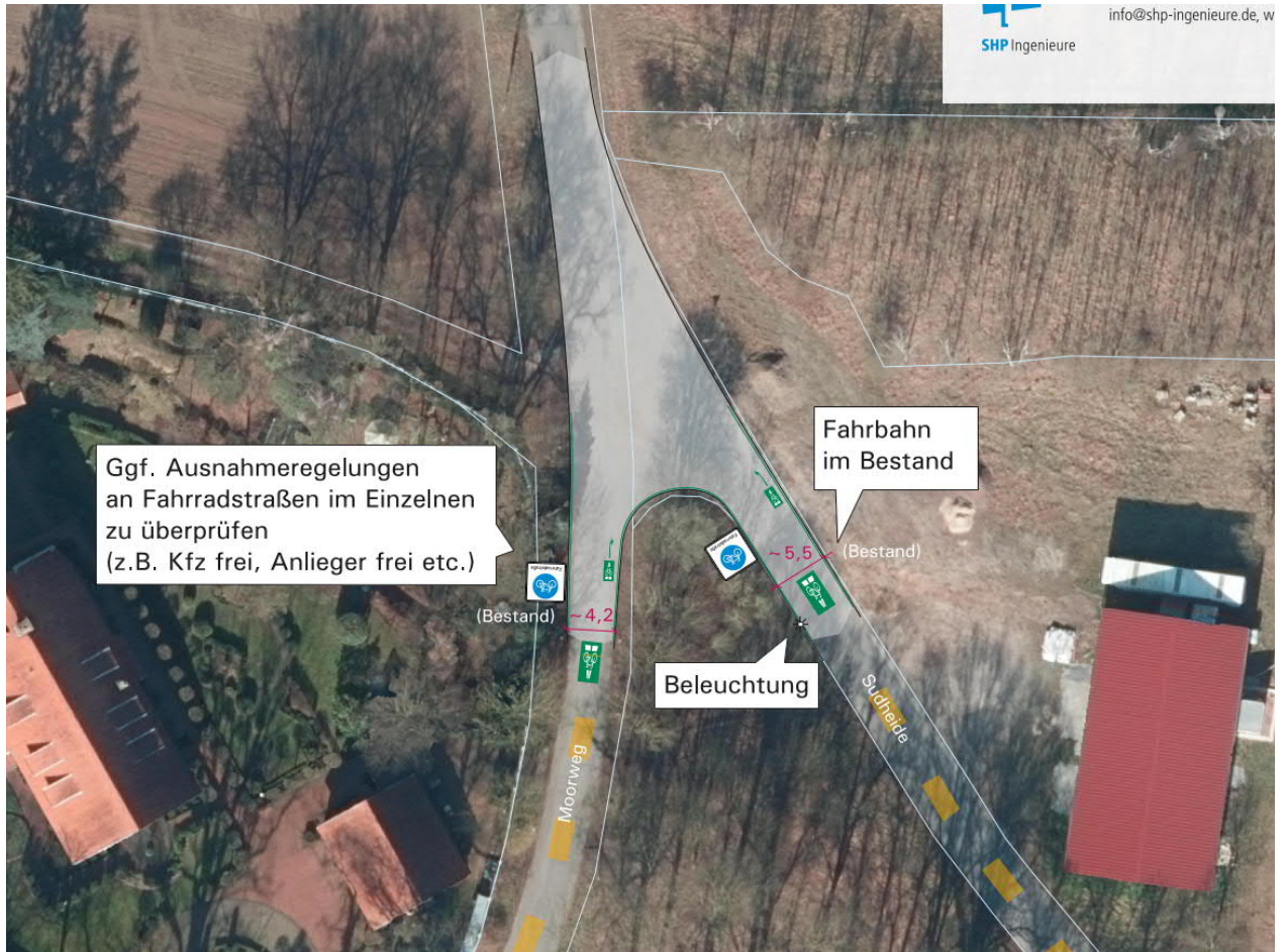
Abb. 29 Ausschnitt Planerische Lösung für den KP Moorweg/Sudheide, Abschnitt RW06/RW07 (nicht maßstäblich, Lageplan maßstabsgetreu und mit weiterführenden Informationen im Anhang)
