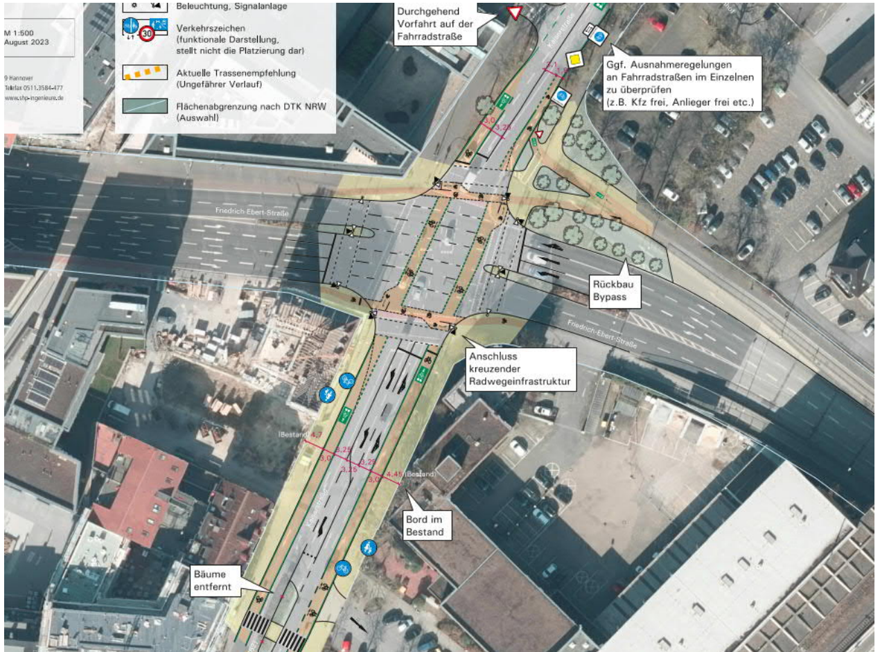
Abb. 34 Ausschnitt Planerische Lösung für den KP Friedrich-Ebert-Straße/Kaiserstraße, GT62/GT07 (nicht maßstäblich, Lageplan maßstabsgetreu und mit weiterführenden Informationen im Anhang)
