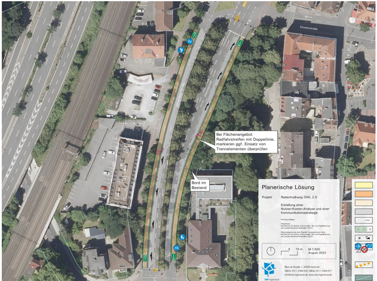
Abb. 43 Ausschnitt Planerische Lösung für einen Abschnitt der Straßen Artur-Ladebeck-Straße/Oberntorwall zwischen Obernstraße und Klosterstraße, BI51 (nicht maßstäblich, Lageplan maßstabsgetreu und mit weiterführenden Informationen im Anhang)
