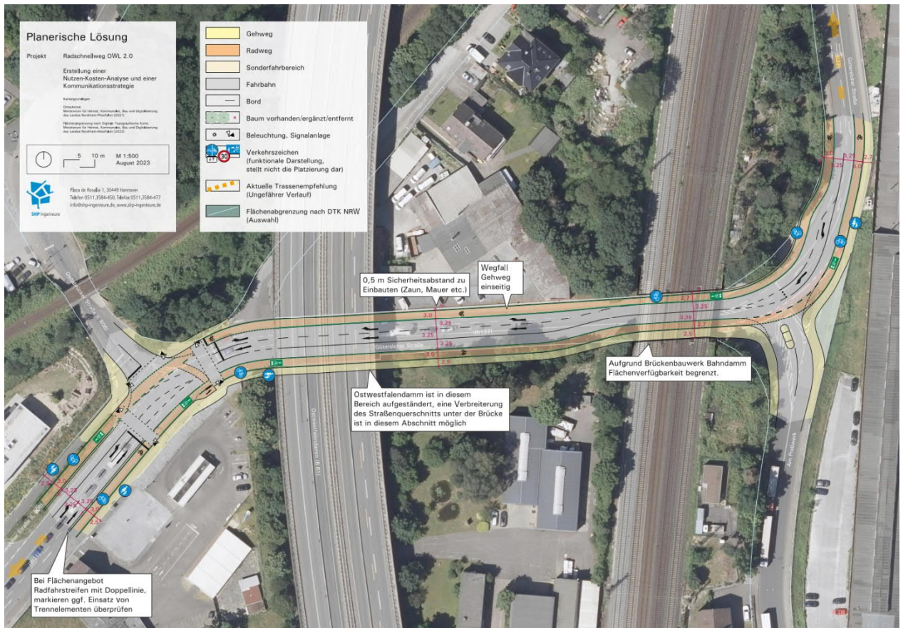
Abb. 40 Ausschnitt Planerische Lösung für einen Abschnitt an der Gütersloher Straße zwischen Osnabrücker Straße und Am Preßwerk, BI21/BI137/BI22 (nicht maßstäblich, Lageplan maßstabsgetreu und mit weiterführenden Informationen im Anhang)
