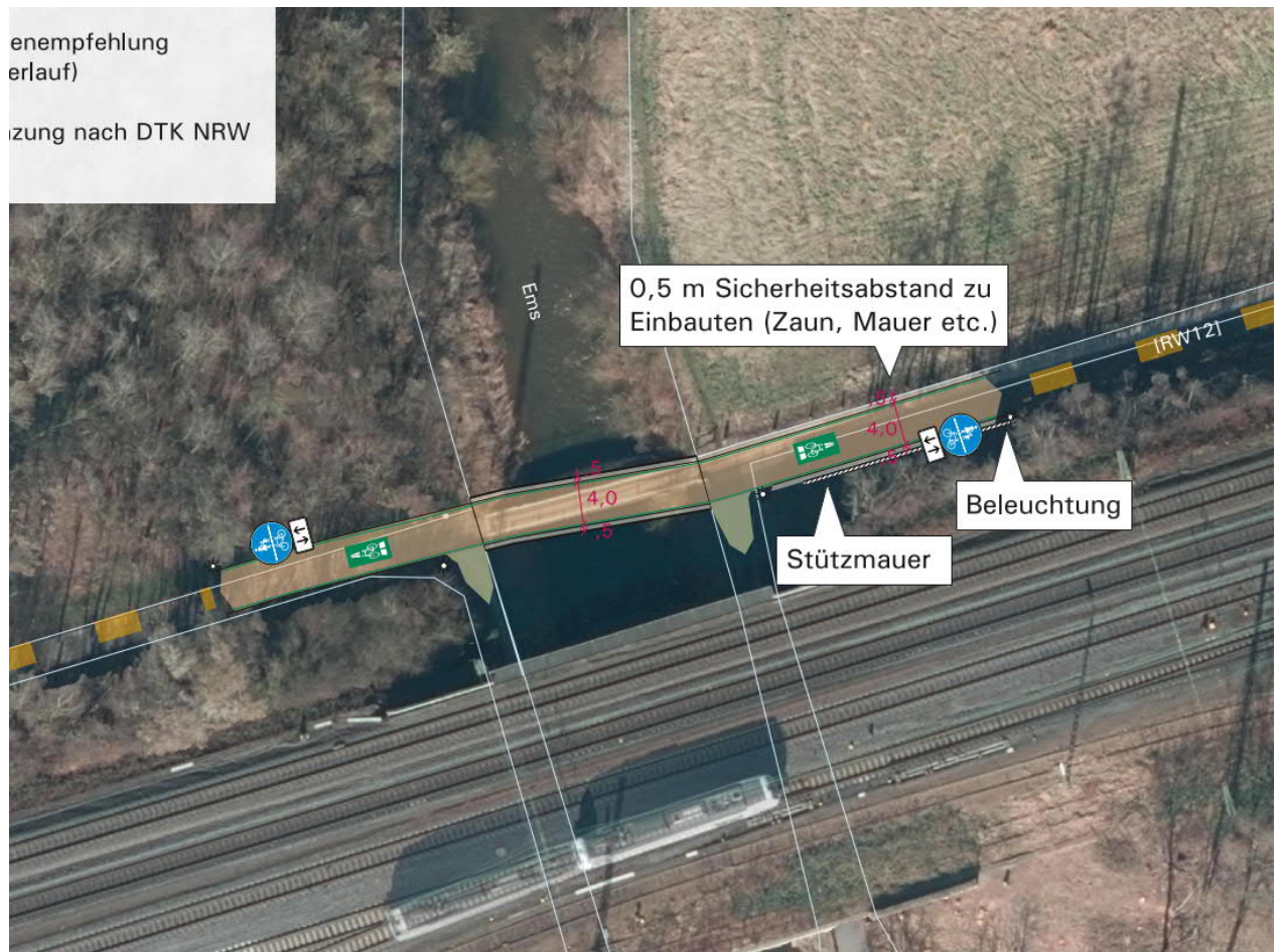
Abb. 27 Ausschnitt Planerische Lösung für ein Brückenbauwerk über die Ems, Abschnitt RW12 (nicht maßstäblich, Lageplan maßstabsgetreu und mit weiterführenden Informationen im Anhang)
