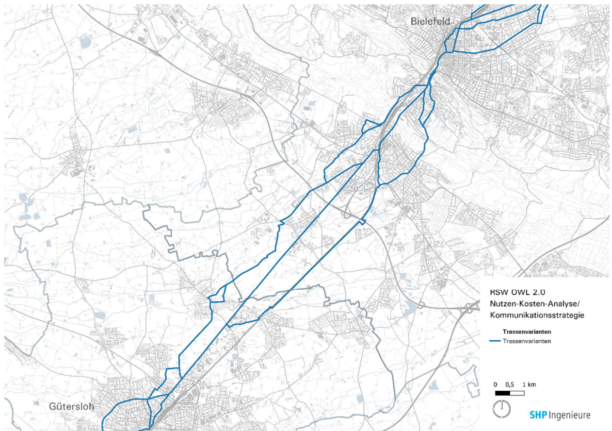
Abb. 3 Trassenvarianten: Abschnitt B
