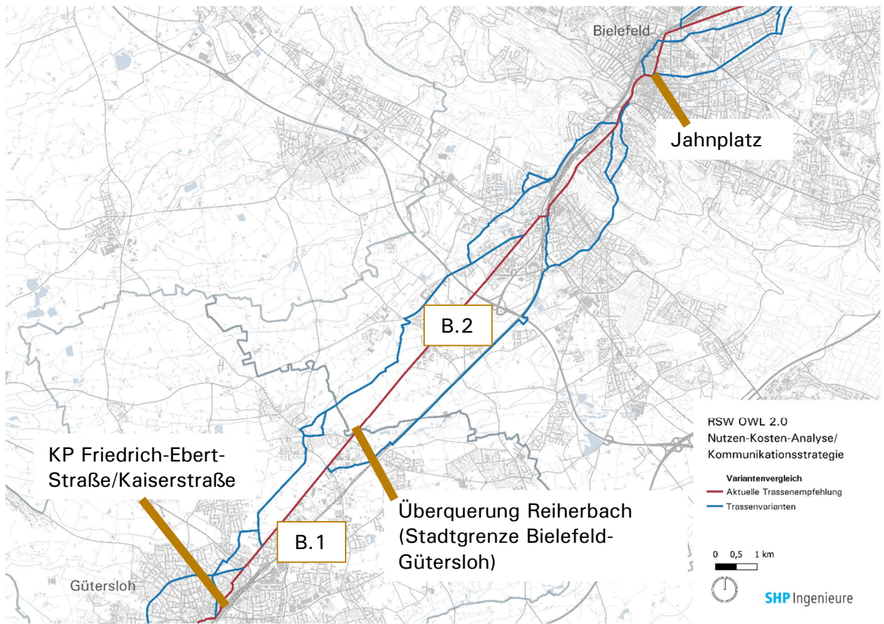
Abb. 35 Aktuelle Trassenempfehlung und Trassenvarianten: Abschnitte B.1 und B.2
