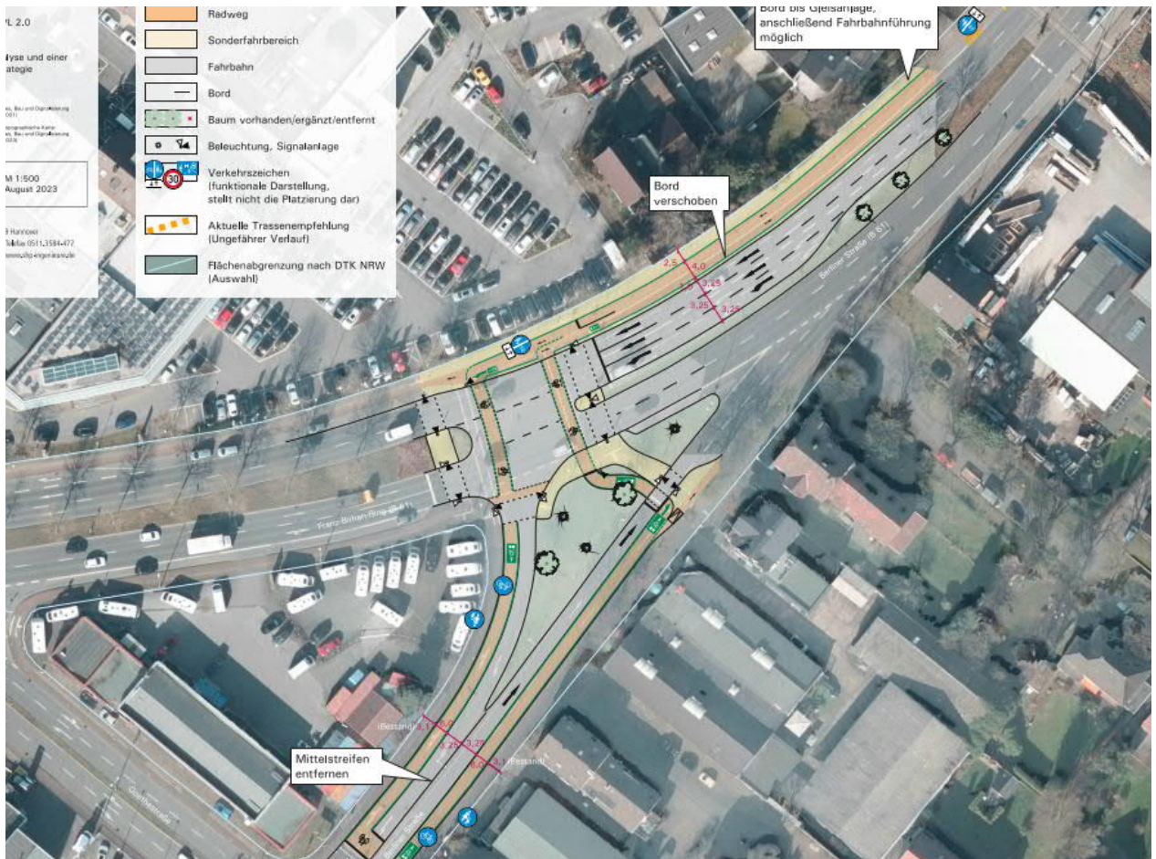
Abb. 36 Ausschnitt Planerische Lösung für den KP Franz-Birkhan-Ring (B 61)/Berliner Straße (B 61)/Berliner Straße, GT08/GT17 (nicht maßstäblich, Lageplan maßstabsgetreu und mit weiterführenden Informationen im Anhang)
