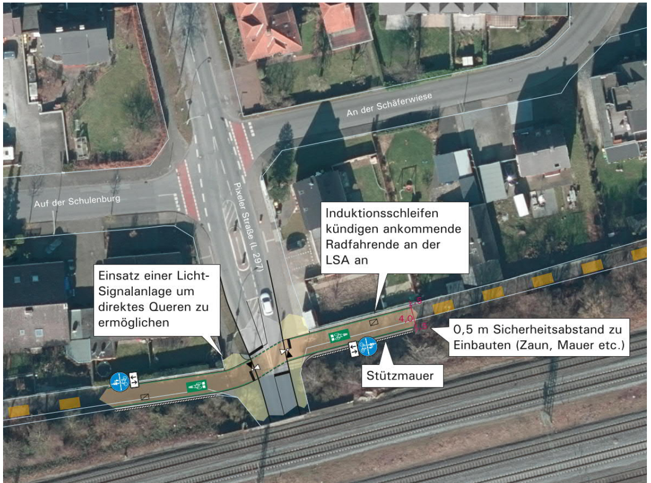
Abb. 26 Ausschnitt Planerische Lösung für den KP Pixeler Straße/Am Bahndamm, Abschnitte RW13/RW14 (nicht maßstäblich, Lageplan maßstabsgetreu und mit weiterführenden Informationen im Anhang)
