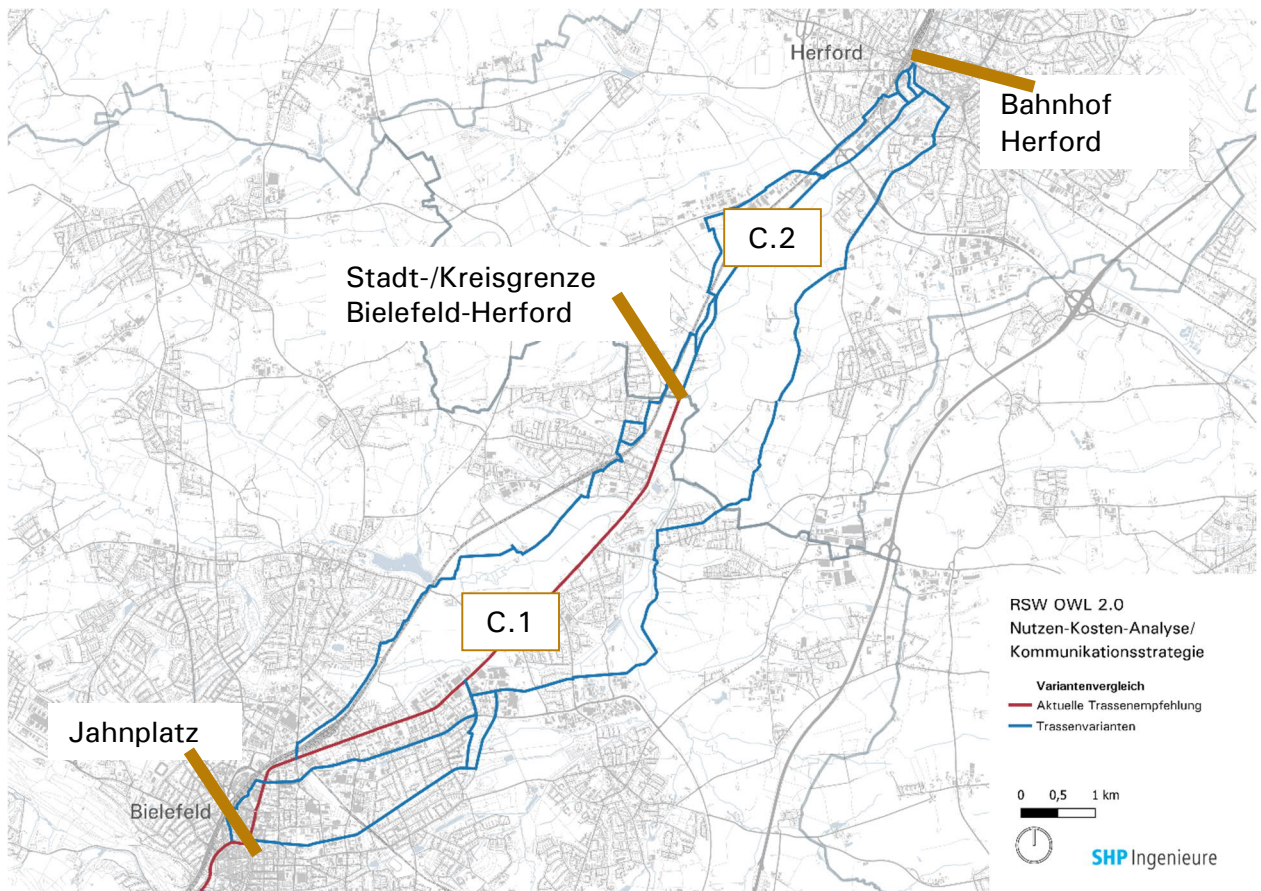
Abb. 44 Aktuelle Trassenempfehlung und Trassenvarianten: Abschnitte C.1 und C.2
