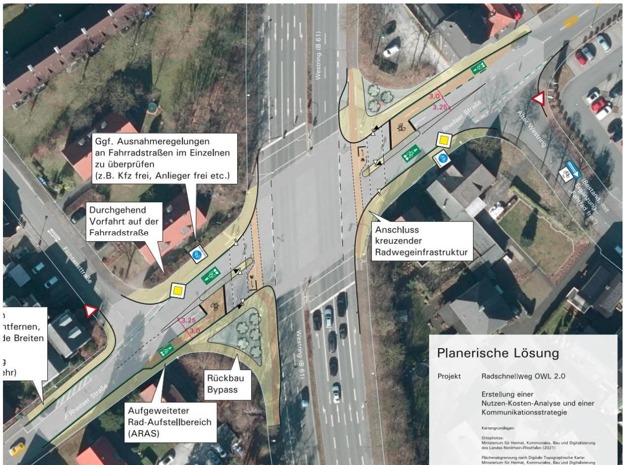
Abb. 30 Ausschnitt Planerische Lösung für den KP Westring/Rhedaer Straße, GT64/GT02 (nicht maßstäblich, Lageplan maßstabsgetreu und mit weiterführenden Informationen im Anhang)
