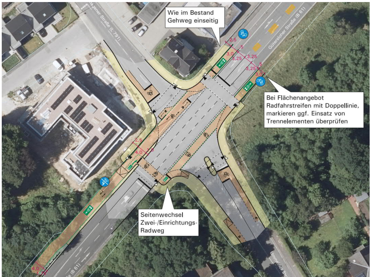
Abb. 39 Ausschnitt Planerische Lösung für einen Abschnitt an der B 61 zwischen Isselhorster Straße und Reiherbach/Stadtgrenze Gütersloh-Bielefeld, BIO1/BI136 (nicht maßstäblich, Lageplan maßstabsgetreu und mit weiterführenden Informationen im Anhang)
