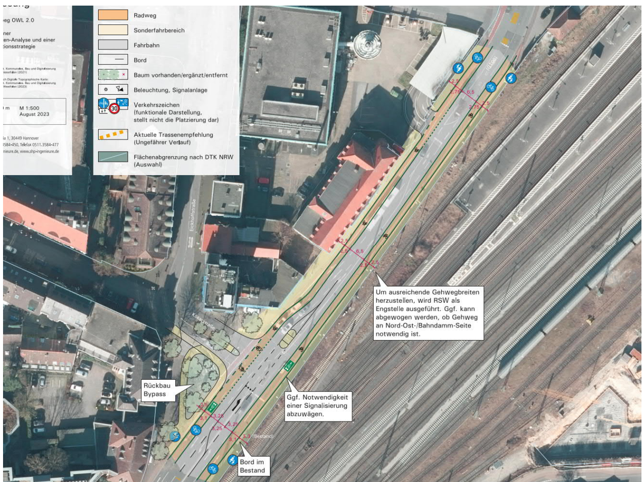
Abb. 33 Ausschnitt Planerische Lösung für die Kaiserstraße zwischen Kirchstraße und ZOB Gütersloh, GT06 (nicht maßstäblich, Lageplan maßstabsgetreu und mit weiterführenden Informationen im Anhang)
