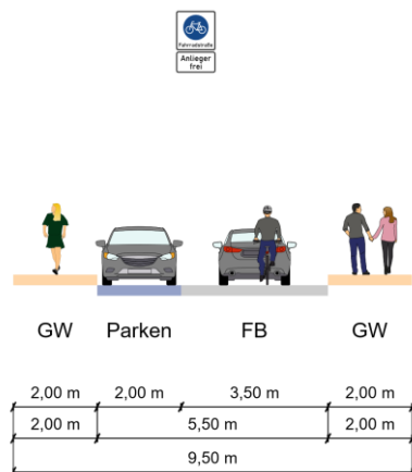
Abbildung 21 Lösungsvorschlag Querschnitt Rolandstraße (G-06)
