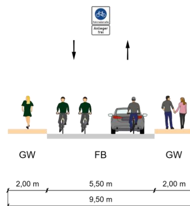
Abbildung 21 Lösungsvorschlag Querschnitt Rolandstraße (G-06)
