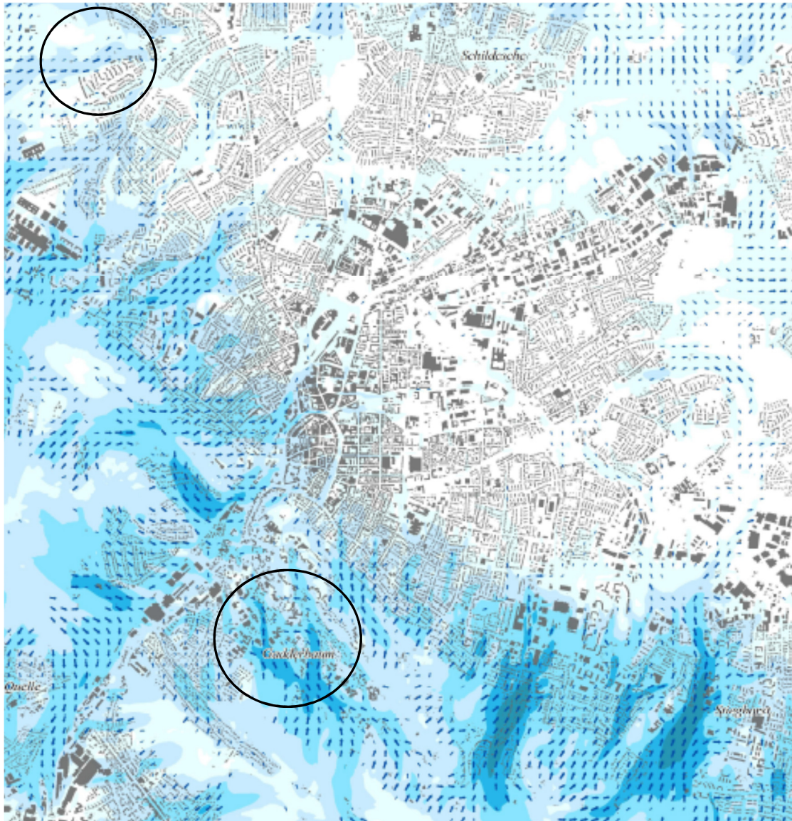
Karte der Kaltluftvolumenstromdichte, Zukunft (Ausschnitt)
